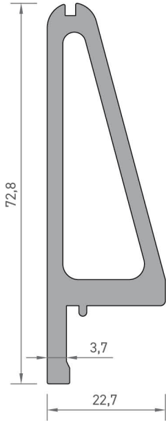
7366 KORKULUK SİSTEM PROFİLİ 1,379 kg/mt
