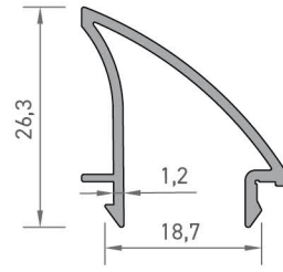
8927 ÇİTA PROFİLİ 0,236 kg/mt
