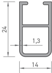
7397 U PROFİLİ 0,248 kg/mt
