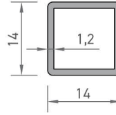
3750 KARE PROFİLİ 0,140 kg/mt
