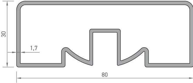
3816 80'LIK ÜST KAPAK PROFİLİ 1,161 kg/mt
