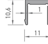
4491 DİKME KAPAK PROFİLİ 0,100 kg/mt
