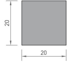
3029 KARE PROFİLİ 1,085 kg/mt
