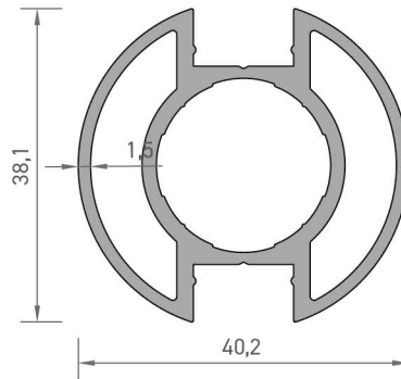
3046 40'LIK DİKME PROFİLİ 0,935 kg/mt
