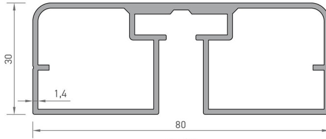
3912 ÜST TUTAMAK PROFİLİ 1,150 kg/mt
