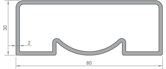
9208 ÜST KAPAK PROFİLİ 1,226 kg/mt
