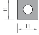
3030 CAM STOP PROFİLİ 0,275 kg/mt
