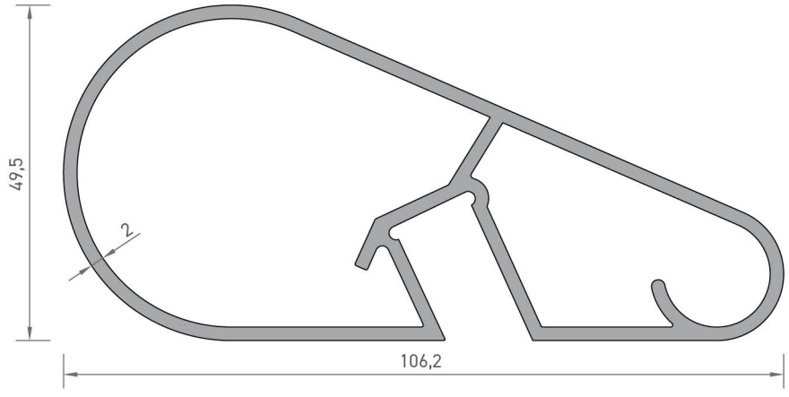
4058 TUTMAK PROFİLİ 1,732 kg/mt
