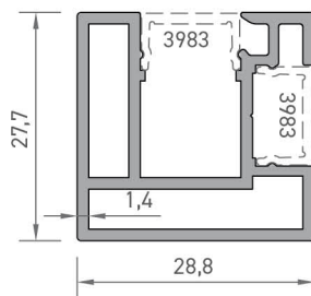
4243 DİKME PROFİLİ 0,536 kg/mt
