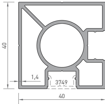
3747 40'LIK DİKME PROFİLİ 1,005 kg/mt
