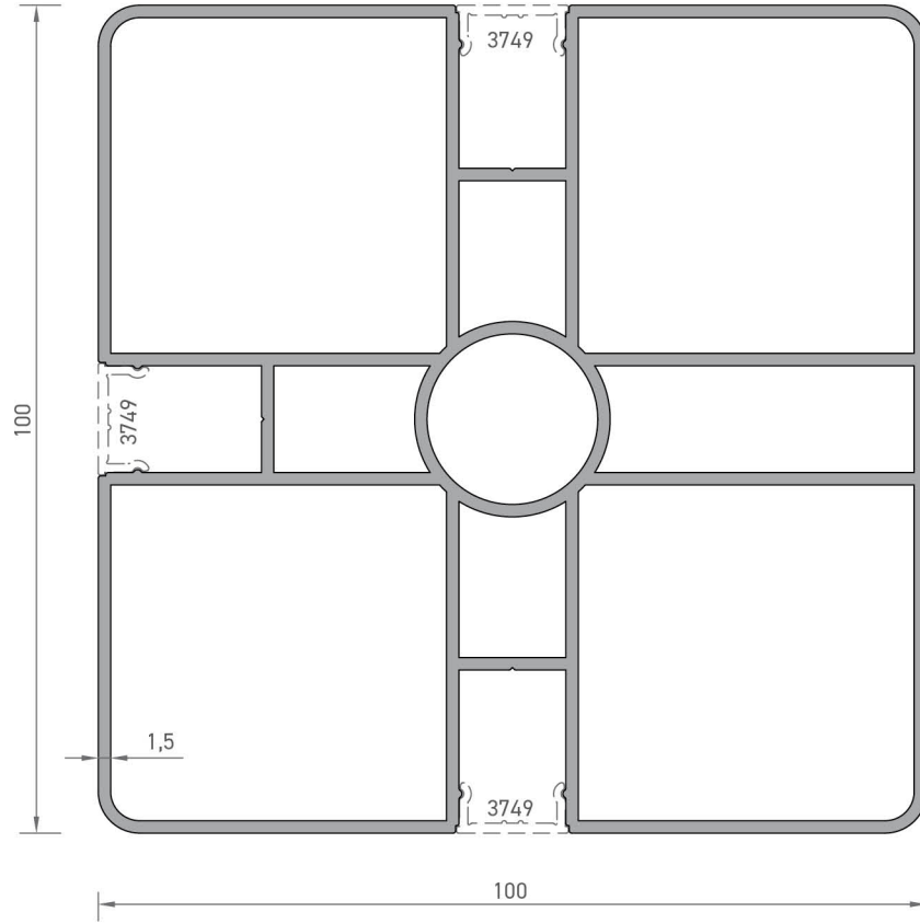
7811 KARE KÜPEŞTE PROFİLİ 3,130 kg/mt
