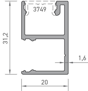
3745 U PROFİLİ 0,382 kg/mt
