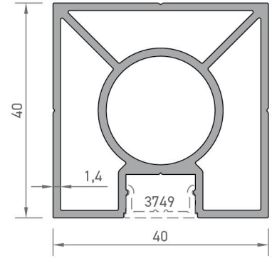
3746 40'LIK DİKME PROFİLİ 1,020 kg/mt
