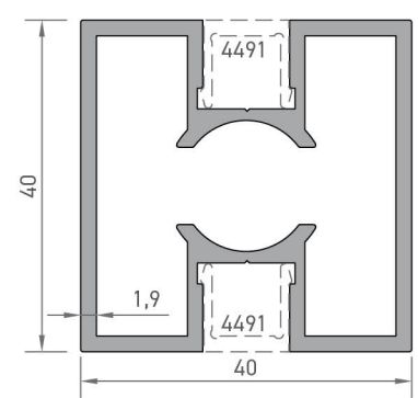
4490 KARE KÜPEŞTE PROFİLİ 1,065 kg/mt
