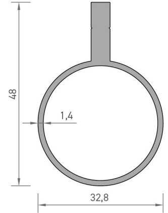
4817 ASKILIK BORU PROFİLİ 0,827 kg/mt
