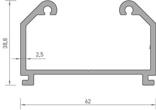
7411 KORKULUK SİSTEM PROFİLİ 1,054 kg/mt
