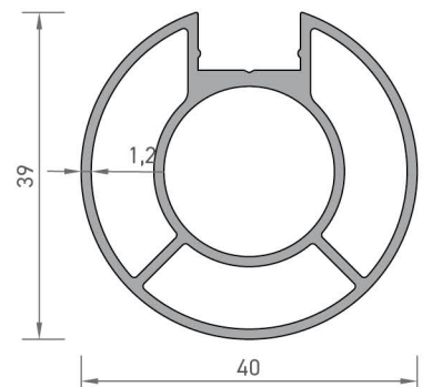
2916 40'LIK DİKME PROFİLİ 0,731 kg/mt
