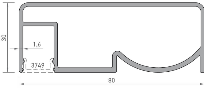
3921 80'LIK ÜST KAPAK PROFİLİ 1,112 kg/mt
