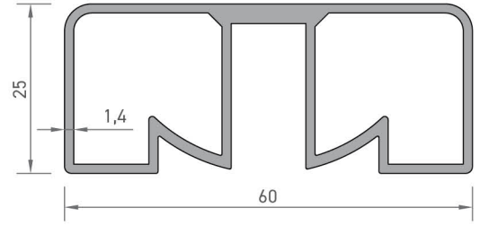
4375 60'LIK ÜST KAPAK PROFİLİ 0,837 kg/mt
