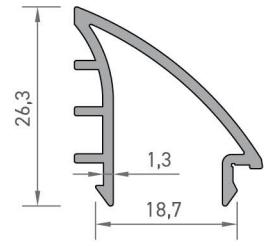
3175 ÇİTA PROFİLİ 0,288 kg/mt
