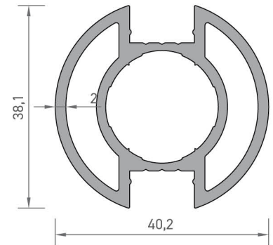
2456 40'LIK DİKME PROFİLİ 1,041 kg/mt
