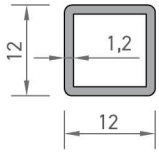
3751 KARE PROFİLİ 0,138 kg/mt
