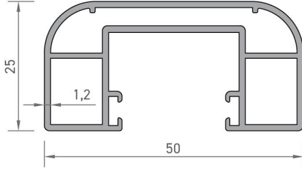
7367 ÜST TUTAMAK PROFİLİ 0,671 kg/mt
