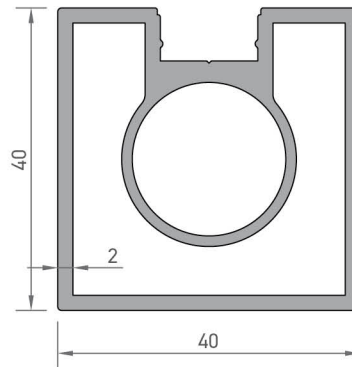
9209 40'LIK DİKME PROFİLİ 1,187 kg/mt
