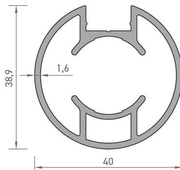
2933 40'LIK DİKME PROFİLİ 0,810 kg/mt
