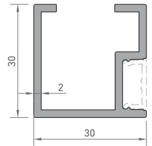
9207 KÜPEŞTE PROFİLİ 0,561 kg/mt
