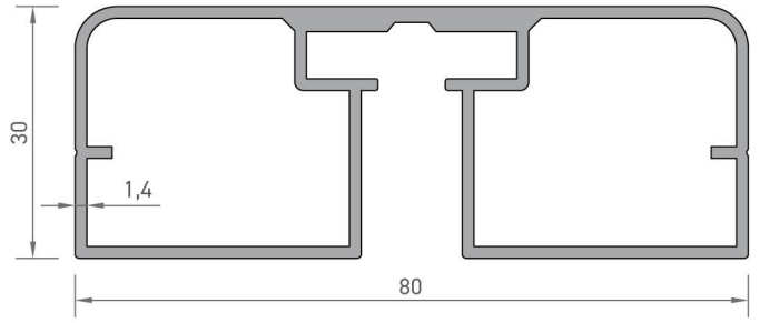
3912 80'LIK ÜST KAPAK PROFİLİ 1,146 kg/mt
