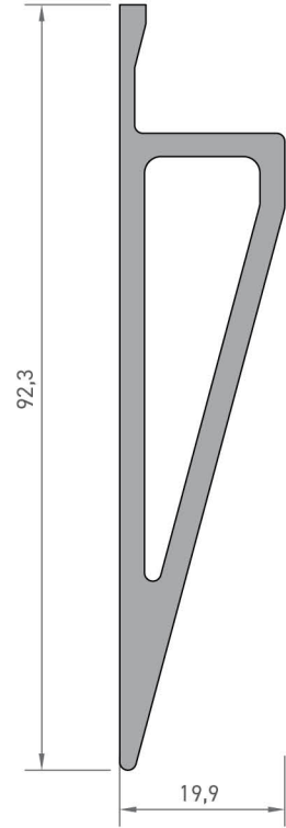
7711 VİDALAMA PROFİLİ 1,393 kg/mt
