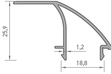
8926 ÇİTA PROFİLİ 0,293 kg/mt
