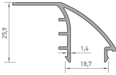
3174 ÇİTA PROFİLİ 0,351 kg/mt
