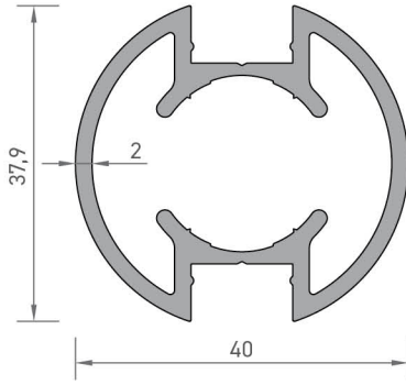
2457 40'LIK DİKME PROFİLİ 0,922 kg/mt
