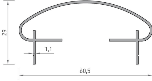
2260 MERDİVEN KÜPEŞTE PROFİLİ 0,415 kg/mt
