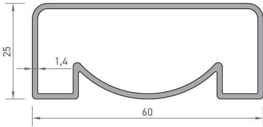
3743 60'LIK ÜST KAPAK PROFİLİ 0,690 kg/mt
