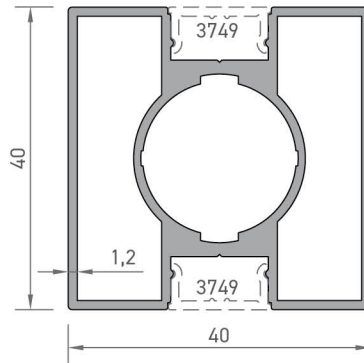
4285 KARE KÜPEŞTE PROFİLİ 0,894 kg/mt
