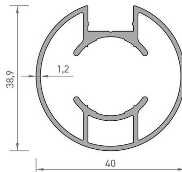
4655 40'LIK DİKME PROFİLİ 0,670 kg/mt
