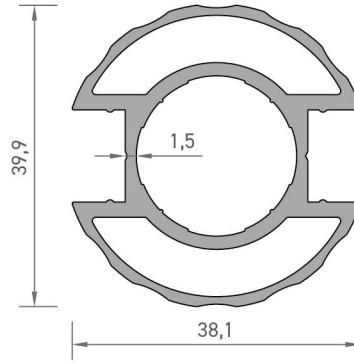
3047 40'LIK DİKME PROFİLİ 0,887 kg/mt
