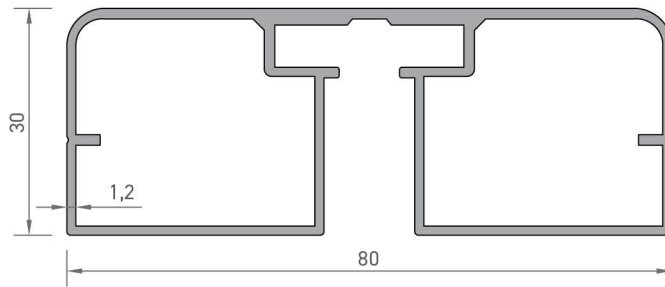
8928 ÜST TUTAMAK PROFİLİ 1,000 kg/mt
