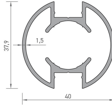
4650 40'LIK DİKME PROFİLİ 0,745 kg/mt
