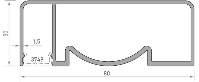
7556 80'LIK ÜST KAPAK PROFİLİ 1,080 kg/mt
