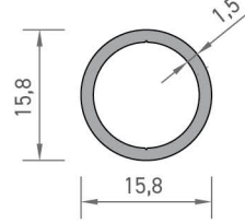
3641 BORU PROFİLİ 0,183 kg/mt
