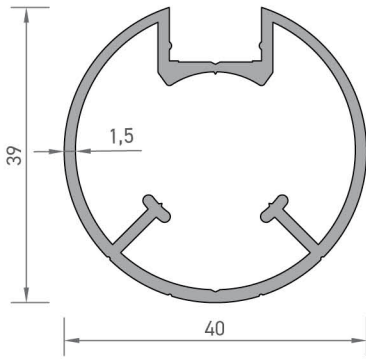
4654 40'LIK DİKME PROFİLİ 0,666 kg/mt
