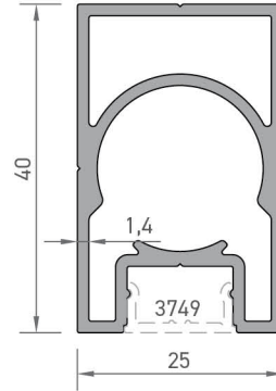
3748 KÜPEŞTE AKSESUAR PROFİLİ 0,721 kg/mt
