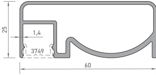
3742 60'LIK ÜST KAPAK PROFİLİ 0,810 kg/mt
