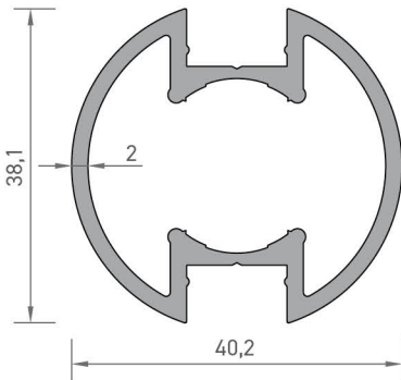
2473 40'LIK DİKME PROFİLİ 0,860 kg/mt
