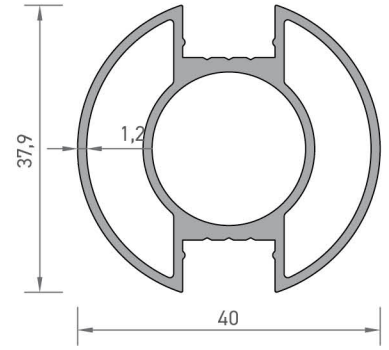
2915 40'LIK DİKME PROFİLİ 0,720 kg/mt
