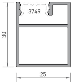
9263 KÜPEŞTE PROFİLİ 0,401 kg/mt
