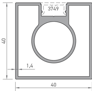
4724 KARE KÜPEŞTE PROFİLİ 0,940 kg/mt
