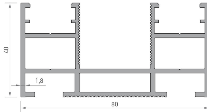
7423 KASA PROFİLİ 1,609 kg/mt
