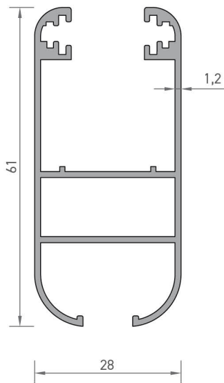
2440 Tek Camlı Kanat Profili 0,710 kg/mt
