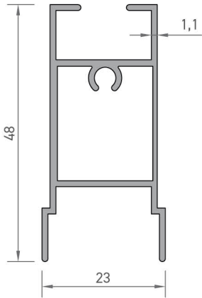
2407 SÜRME KANAT ALT PROFİLİ 0,465 kg/mt
