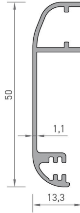
2443 GENİŞ PERVAZ PROFİLİ 0,305 kg/mt
