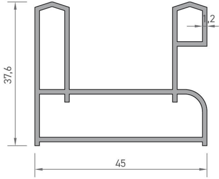
2444 SÜRME KASA PROFİLİ 0,695 kg/mt
