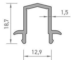
4211 ORTA ADAPTÖR PROFİLİ 0,220 kg/mt
