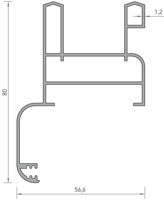
2425 PERVAZLI SÜRME KASA PROFİLİ 0,980 kg/mt
