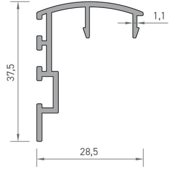
2441 SÜRME KENET PROFİLİ 0,335 kg/mt
