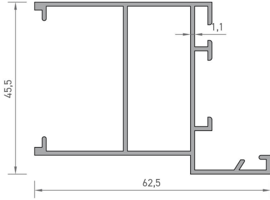
2433 DAR AÇIK KASA PROFİLİ 0,700 kg/mt
