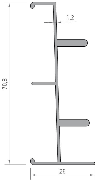
2403 SÜRME KASA ALT PROFİLİ 0,600 kg/mt
