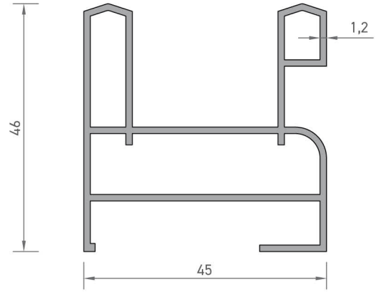
2438 SÜRME KASA PROFİLİ 0,785 kg/mt
