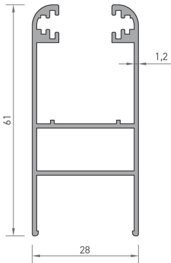
2439 Isi Camlı Kanat Profili 0,680 kg/mt
