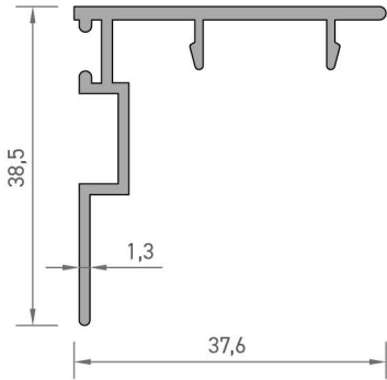
2424 SÜRME KENET PROFİLİ 0,375 kg/mt
