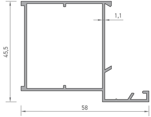
2429 GENİŞ KASA PROFİLİ 0,600 kg/mt
