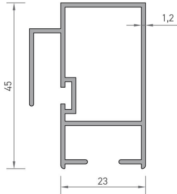
2405 SÜRME KANAT ORTA PROFİLİ 0,565 kg/mt
