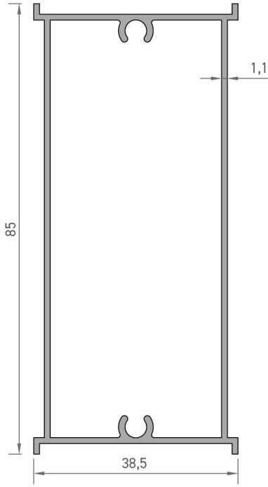
2431 Panjur Kayıt Profili 0,785 kg/mt
