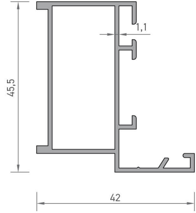
2426 DAR KASA PROFİLİ 0,555 kg/mt
