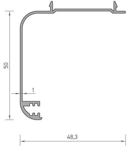
2442 GENİŞ PERVAZ PROFİLİ 0,360 kg/mt
