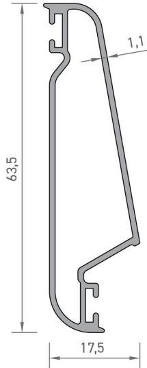
2445 PANJUR KANAT PROFİLİ 0,480 kg/mt
