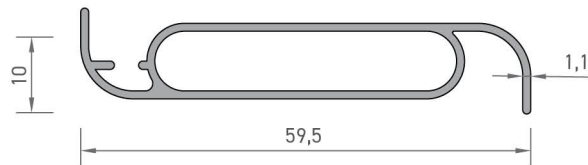
2434 PANJUR YAPRAK PROFİLİ 0,390 kg/mt
