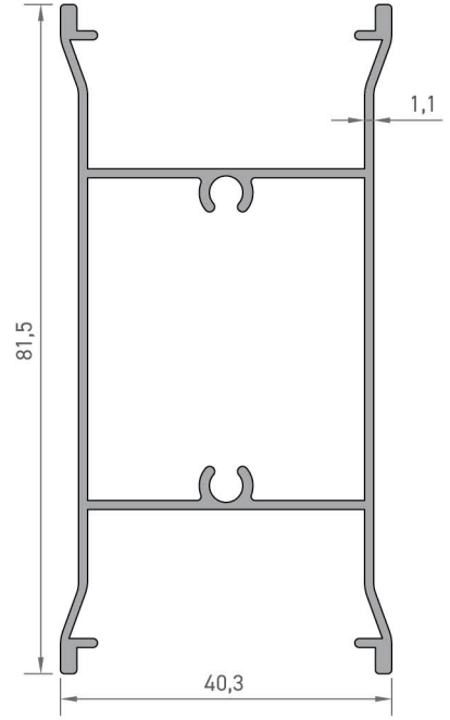
2437 Panjur Kayıt Profili 0,820 kg/mt
