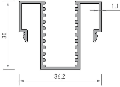
2447 PANJUR ADAPTÖR PROFİLİ 0,490 kg/mt
