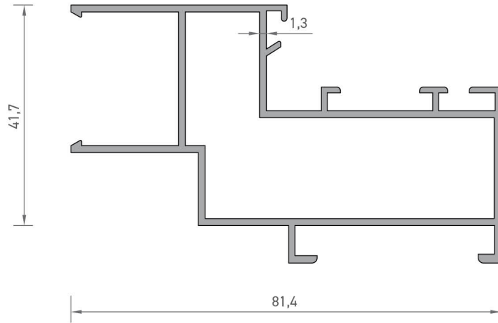
2428 2'Lİ AÇILIR KASA PROFİLİ 1,030 kg/mt
