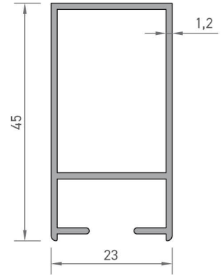
2404 SÜRME KANAT YAN PROFİLİ 0,450 kg/mt
