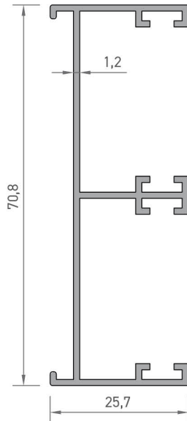
2401 SÜRME KASA ÜST PROFİLİ 0,560 kg/mt
