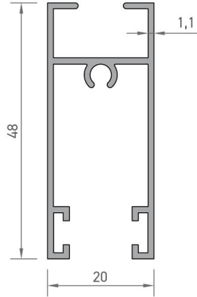
2406 SÜRME KANAT ÜST PROFİLİ 0,460 kg/mt
