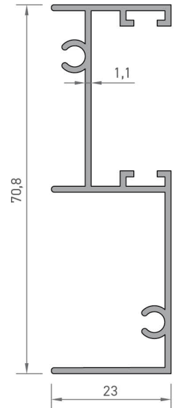
2402 SÜRME KASA ÜST PROFİLİ 0,545 kg/mt
