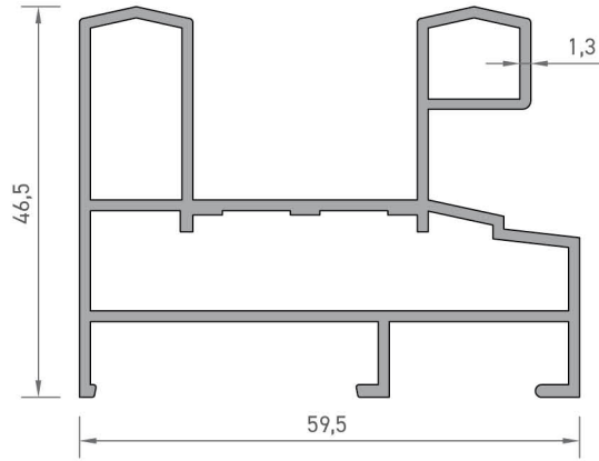
2422 SÜRME KASA PROFİLİ 1,030 kg/mt
