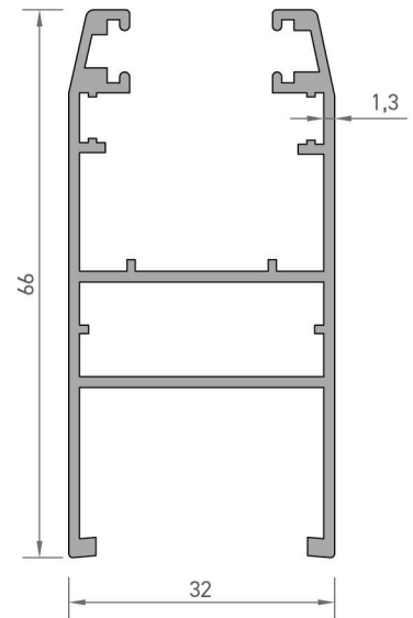
2423 Sürme Kanat Profili 0,850 kg/mt
