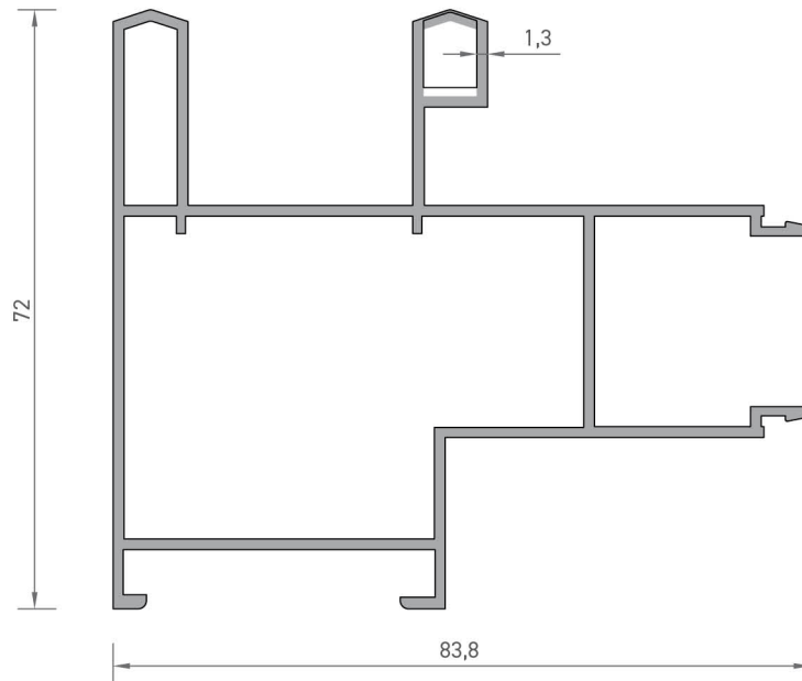
2427 2'Lİ SÜRME KASA PROFİLİ 1,310 kg/mt
