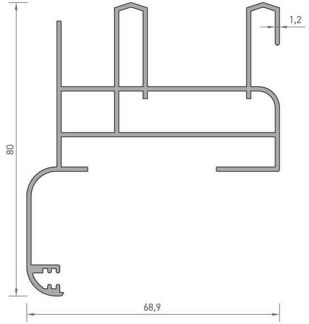
4205 PERVAZLI KASA PROFİLİ 1,200 kg/mt
