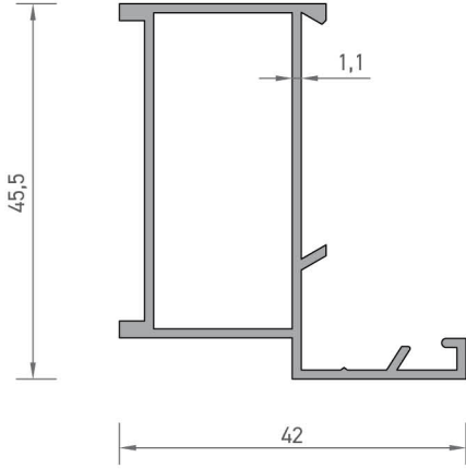
2432 DAR KASA PROFİLİ 0,505 kg/mt
