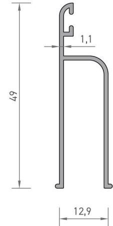
2446 PANJUR KANAT BİTİŞ PROFİLİ 0,305 kg/mt
