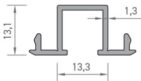
4217 TEK CAM ADAPTÖR PROFİLİ 0,225 kg/mt
