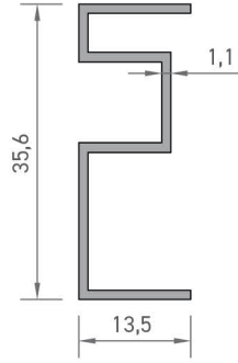
2435 PNJUR YAN PROFİLİ 0,245 kg/mt
