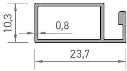
2043 MİNİ SİNEKLİK PROFİLİ 0,154 kg/mt
