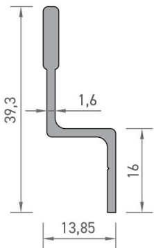
2054 SİNEKLİK RAY PROFİLİ 0,268 kg/mt
