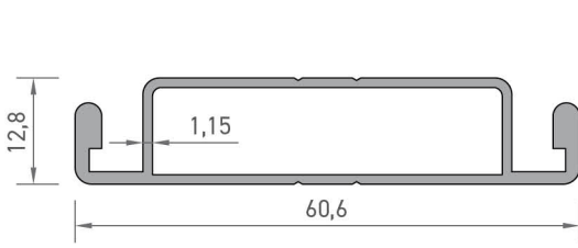
2870 SİNEKLİK KANAT PROFİLİ 0,514 kg/mt
