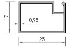
2051 PENCERE SİNEKLİK PROFİLİ 0,226 kg/mt
