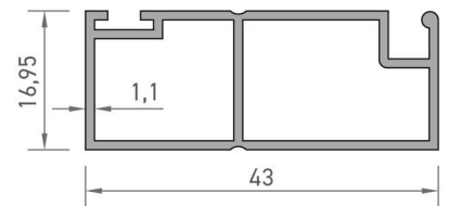
2835 KAPI SİNEKLİK PROFİLİ 0,422 kg/mt
