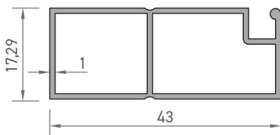
2050 KAPI SİNEKLİK PROFİLİ 0,371 kg/mt
