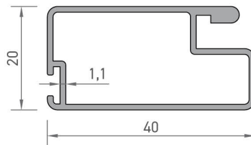
2833 SİNEKLİK KANAT PROFİLİ 0,412 kg/mt
