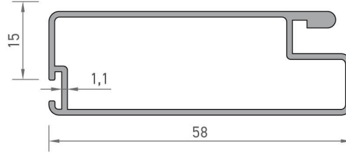
2861 SİNEKLİK KANAT PROFİLİ 0,520 kg/mt
