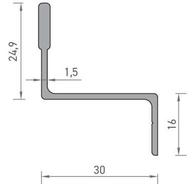
2029 SİNEKLİK RAY PROFİLİ 0,328 kg/mt
