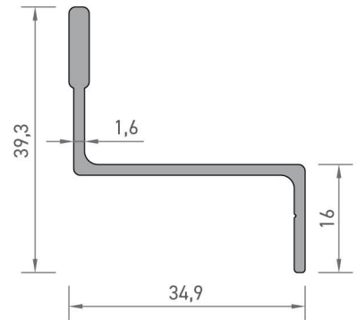
2076 SİNEKLİK RAY PROFİLİ 0,359 kg/mt
