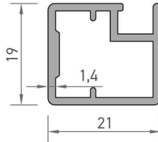
2843 SİNEKLİK KANAT PROFİLİ 0,337 kg/mt
