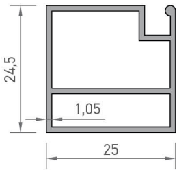
2910 PENCERE SİNEKLİK KANAT PROFİLİ 0,355 kg/mt
