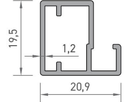
3298 SİNEKLİK KANAT PROFİLİ 0,274 kg/mt
