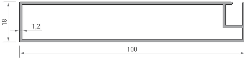
3147 SİNEKLİK KANAT PROFİLİ 0,795 kg/mt
