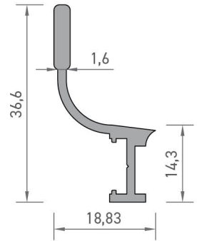
3320 SİNEKLİK RAY PROFİLİ 0,290 kg/mt
