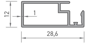
3365 SİNEKLİK PROFİLİ 0,232 kg/mt
