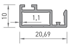
3364 SİNEKLİK PROFİLİ 0,179 kg/mt
