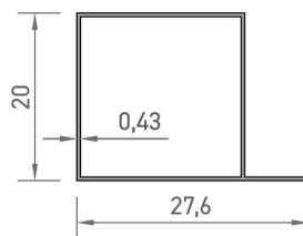
7739 İÇE AÇILIR SİNEKLİK KASA PROFİLİ 0,396 kg/mt
