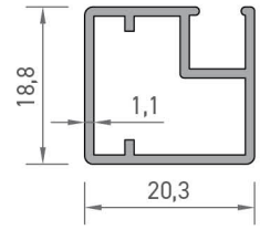
2858 SİNEKLİK PROFİLİ 0,255 kg/mt
