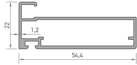
3413 SİNEKLİK PROFİLİ 0,559 kg/mt
