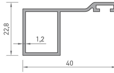
2083 FİTİLLİ SİNEKLİK KASA PROFİLİ 0,328 kg/mt
