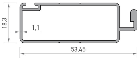
2862 SİNEKLİK KANAT PROFİLİ 0,463 kg/mt
