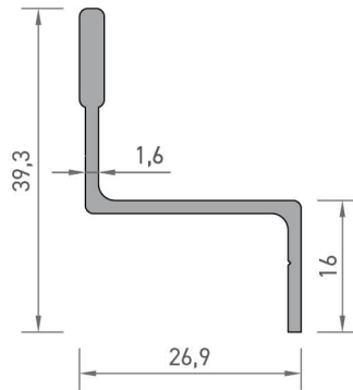
2026 SİNEKLİK RAY PROFİLİ 0,325 kg/mt
