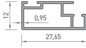
3057 SİNEKLİK KANAT PROFİLİ 0,224 kg/mt
