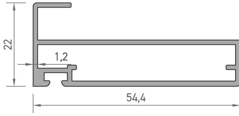
3288 SİNEKLİK PROFİLİ 0,554 kg/mt
