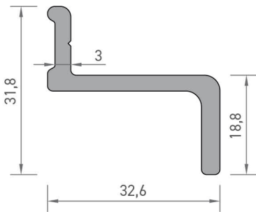
2055 SİNEKLİK RAY PROFİLİ 0,528 kg/mt
