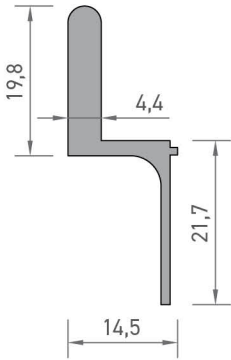
1962 SİNEKLİK RAY PROFİLİ 0,355 kg/mt
