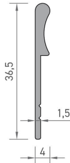
3428 SİNEKLİK RAY PROFİLİ 0,119 kg/mt
