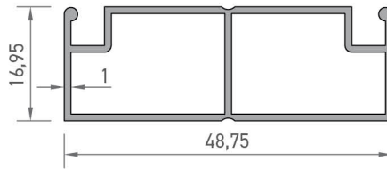
3321 KAPI SİNEKLİK PROFİLİ 0,423 kg/mt
