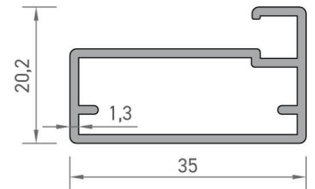
2099 SİNEKLİK KANAT PROFİLİ 0,396 kg/mt
