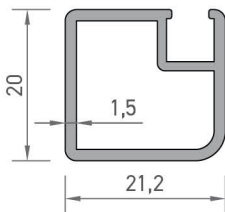
2960 SİNEKLİK KANAT PROFİLİ 0,322 kg/mt
