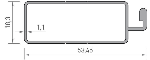
2869 SİNEKLİK KANAT PROFİLİ 0,447 kg/mt
