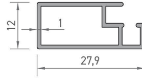
2871 SİNEKLİK KANAT PROFİLİ 0,222 kg/mt
