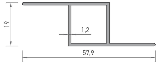
2049 İÇE AÇILIR SİNEKLİK KASA PROFİLİ 0,354 kg/mt
