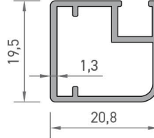
3223 SİNEKLİK KANAT PROFİLİ 0,270 kg/mt
