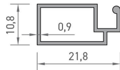
2544 MİNİ SİNEKLİK PROFİLİ 0,161 kg/mt
