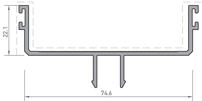
Eşiksiz Kasa Kapak Profili Threshold Frame Cover Profile
