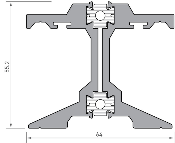
Eşiksiz Kasa Adaptör Profili Threshold Frame Adapter Profile
