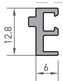
Cam Çıtası Profili Glazing Bead Profile
