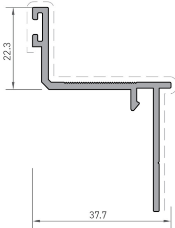
Eşiksiz Kasa Kapak Profili Threshold Frame Cover Profile
