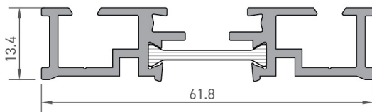
Kanat Adaptör Profili Sash Adapter Profile
