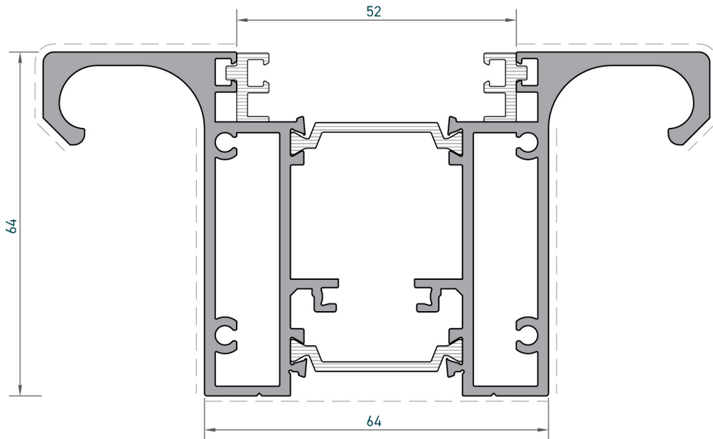
Kulplu Kanat Profili Handle Sash Profile
