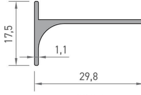
3443 T PROFİLİ 0,166 kg/mt
