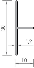
4516 T PROFİLİ 0,125 kg/mt
