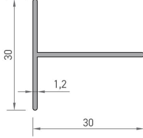
2190 T PROFİLİ 0,190 kg/mt
