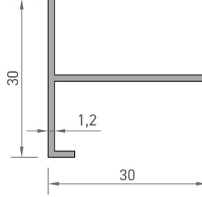
7257 T PROFİLİ 0,203 kg/mt
