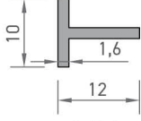
8077 T PROFİLİ 0,089 kg/mt
