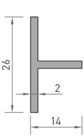
4423 T PROFİLİ 0,208 kg/mt
