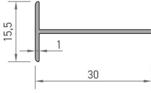
3444 T PROFİLİ 0,120 kg/mt
