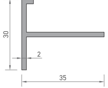
2528 T PROFİLİ 0,358 kg/mt
