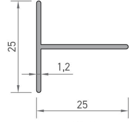
2156 T PROFİLİ 0,158 kg/mt
