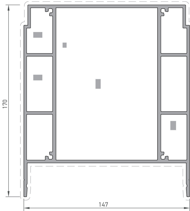
Dikme Profili / Column Profile
