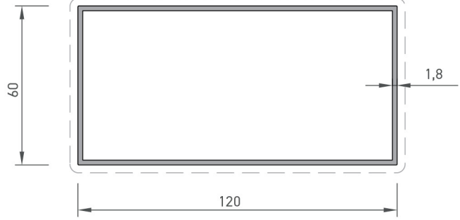
Kutu Profili / Box Profile
