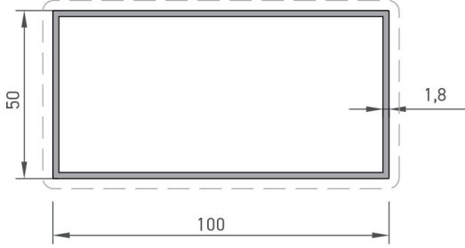
Kutu Profili / Box Profile
