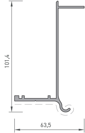
Açık Ayar Profili Angle Adjustment Profile
