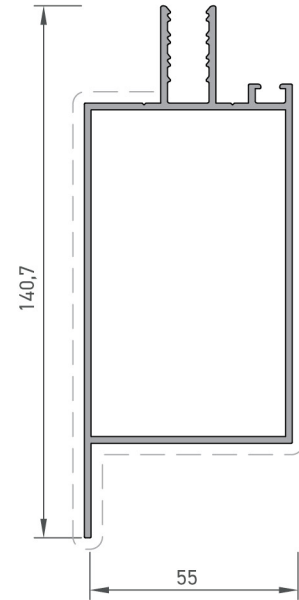
Bitiş Griyaj Profili / End Mullion Profile
