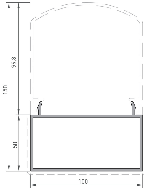
Dikme Profili / Column Profile
