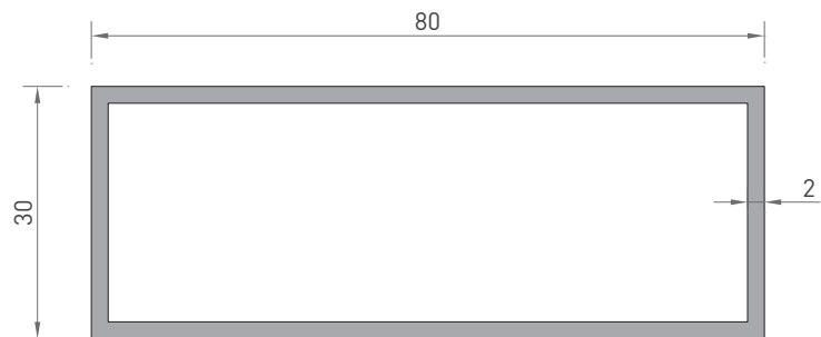
2211 30 x 80 KUTU PROFİL 1.150 kg/mt
