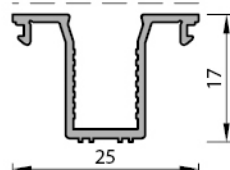
8 MM CAM ÇİTA PROFİL V.ES.115 0.178 kg/mt
