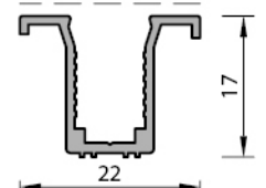
8 MM CAM ÇİTA PROFİL V.ES.116 0.169 kg/mt
