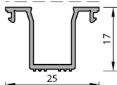
10 MM CAM ÇİTA PROFİL V.ES.104 0.176 kg/mt
