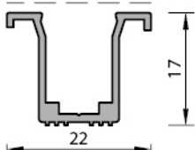
10 MM CAM ÇİTA PROFİL V.ES.103 0.174 kg/mt
