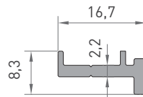
4150 SABİTLEME TAKOZU 0.145 kg/mt
