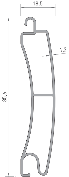
2213 PALET PROFİL 0.705 kg/mt
